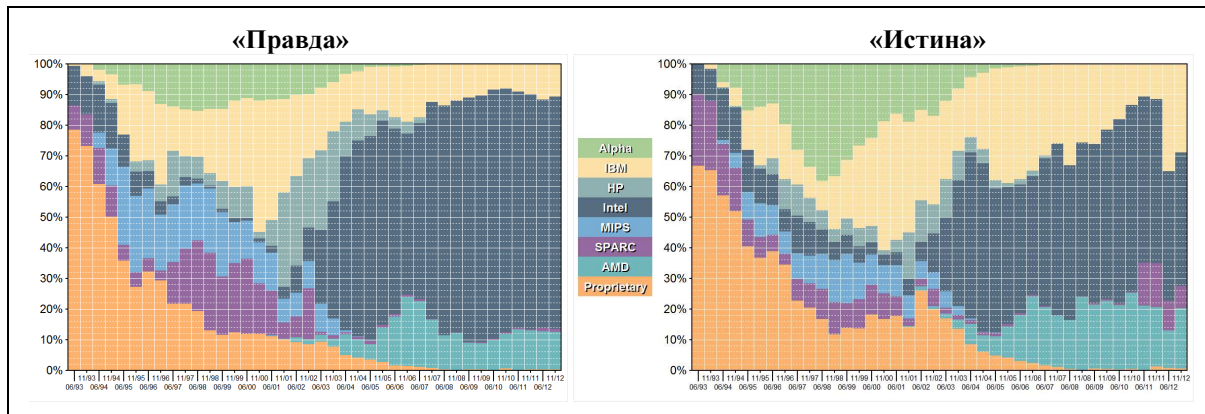
Рис. 8. Доли различных технологий процессоров, используемых в суперкомпьютерах по данным всех 40 редакций рейтинга Top500 (от июня 1993 года по ноябрь 2012 года). Слева доли «в штуках» (доли от общего числа суперкомпьютеров), справа истинные доли (доли в Linpack-производительности)
