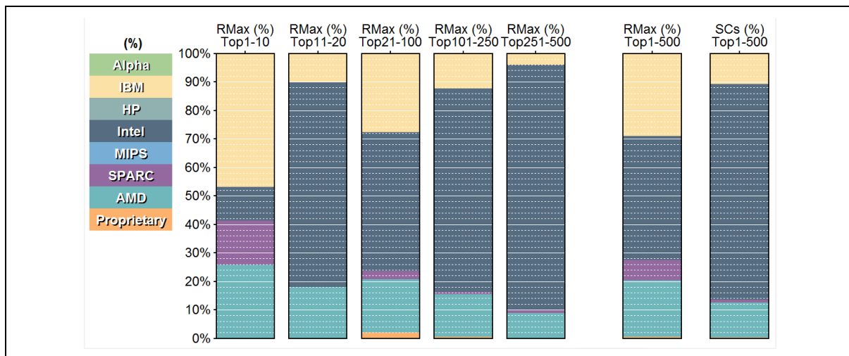
Рис. 9. Распределение технологий процессоров по уровням Top1–10, Top11–20, Top21–100, Top101–250, Top251–500. По данным Top500 за ноябрь 2012 года
