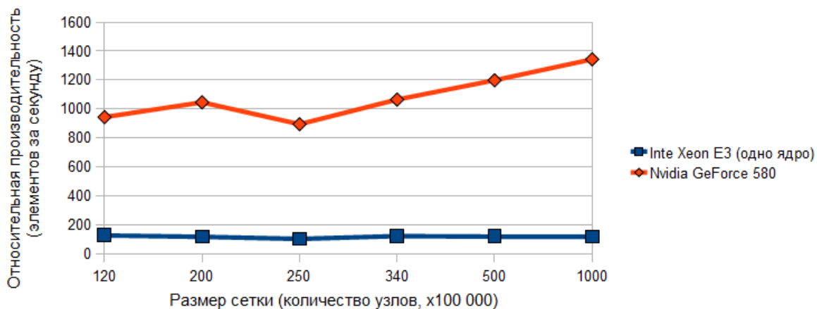
Рис. 3. Производительность версий пакета в зависимости от размера сеток.
