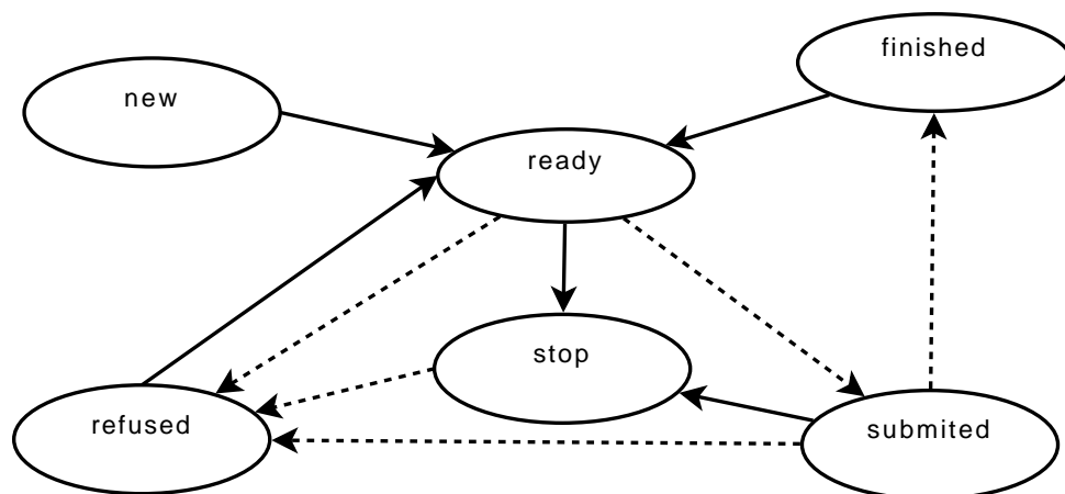
Рис. 1. Граф переходов между значениями статуса задачи. Сплошной стрелкой обозначены переходы, которые пользователь может произвести самостоятельно. Разрывной стрелкой – переходы, которые делаются автоматически.
